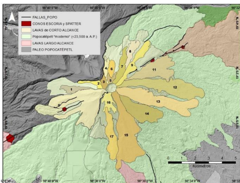
Figura 27. Flujos de lava con origen en el cráter central o en edificios adventicios que conforman la parte cimera del volcán "joven" Popocatepetl. Se desconoce la geocronología del emplazamiento de estos flujos, pero se considera que todos ellos son posteriores a los ~14,100 años A. P. edad de la erupción pliniana "PWA o Tutti-Frutti", que destruyó la parte cimera del cráter y dejó como remanente las lavas del Fraile al SW (sector 0 en amarillo en la figura). lavas del Fraile al SW (sector 0 en amarillo en la figura).
