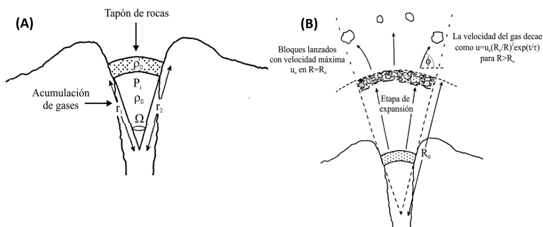
Figura 65. Diagrama del modelo de Fagents y Wilson (1993). En el inciso (A) se muestra la geometría que consideraron para resolver la ecuación de movimiento y en (B) se muestra la expansión de roca y gas hasta la distancia R_0 en la cual los bloques son lanzados.
