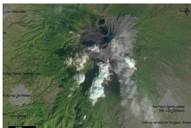
Figura 55. Imagen Landsat 7 TM falso color 1,2,3 del 11 de enero de 1995, se observa una columna de ceniza dirigiéndose al sureste.
