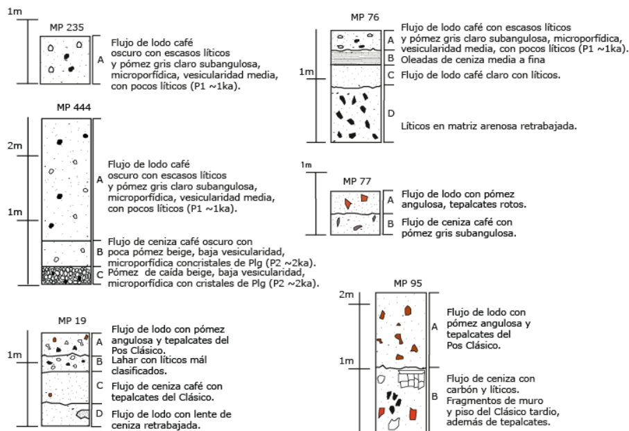
Figura 34. Columnas estratigráficas de la zona Nexapa-Amecameca.
