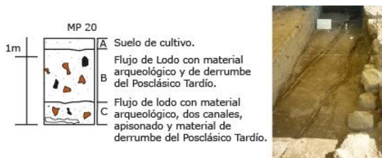
Figura 48. Columna estratigráfica del Sitio Nepantla, se observan sistema de canales.
