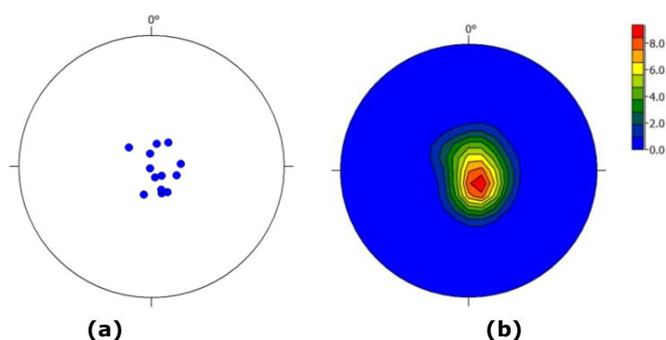
Figura 8. Diagramas estereográficos de las foliaciones en el domo de Tlamacas. En a se muestran los polos (13 datos) de dichas foliaciones, y aunque el número de mediciones es pequeño, si indican tendencia a tener echados suaves, preferencialmente al NNW y SSE. En b, se muestra la distribución estadística de esos polos, confirmando las observaciones de a.
