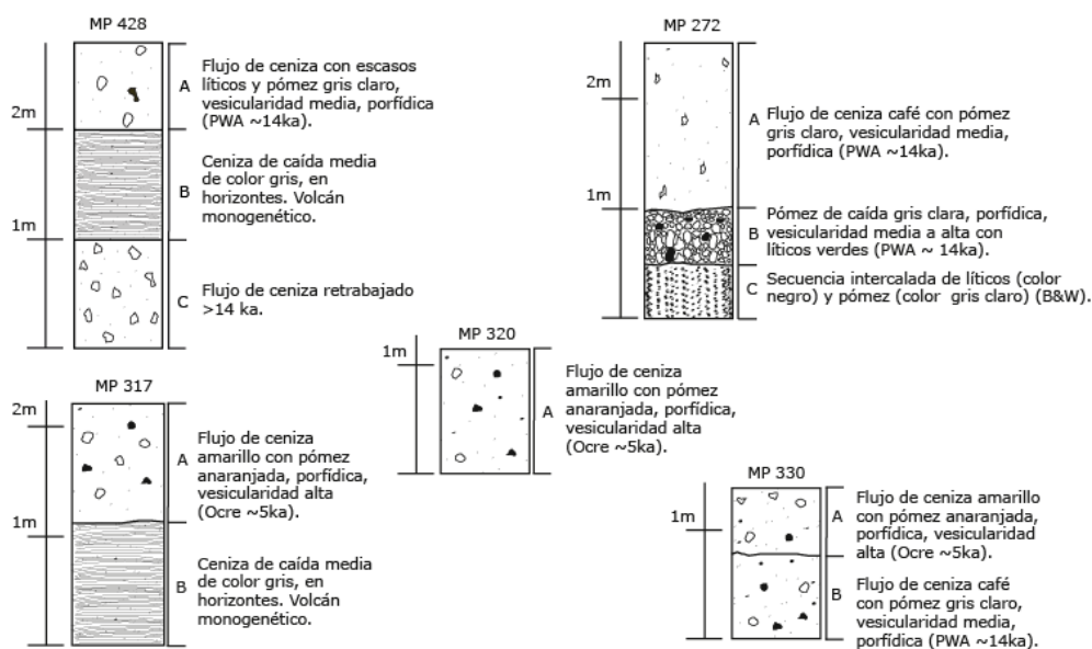
Figura. 40. Secciones estratigráficas de la zona Cuijingo-Tenango.
