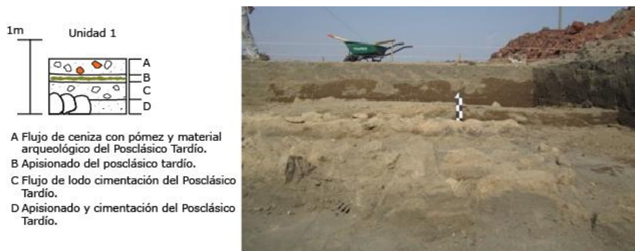
Figura 43. Flujos de lodo entre los apisonados.
