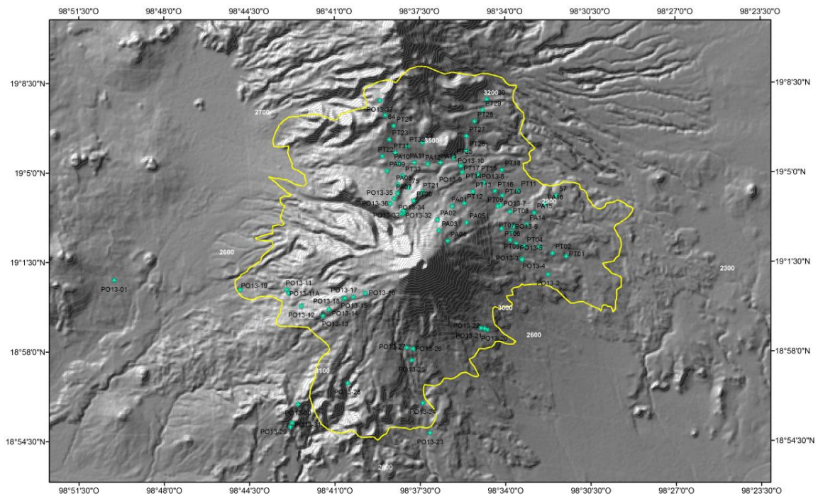
Figura 51. Modelo digital de elevación del volcán Popocatepetl donde se muestra con línea amarilla el límite de la zona donde están distribuidas las Cenizas Negras. En verde, los puntos de verificación.
