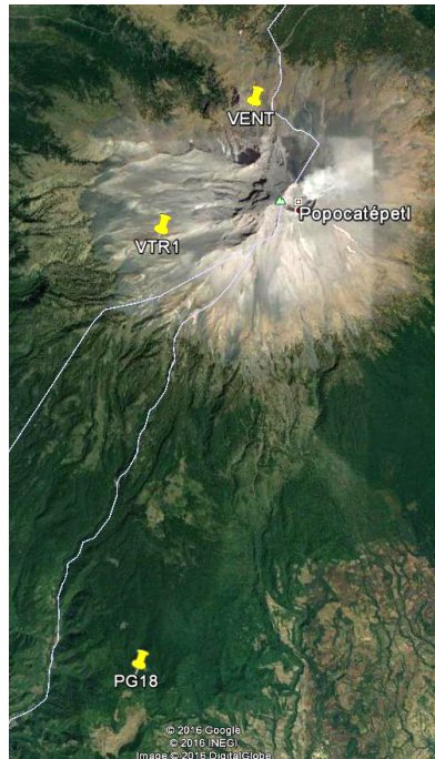
Figura 16. Estaciones del Volcán Ventorrillo. Imagen de Google Earth®.
