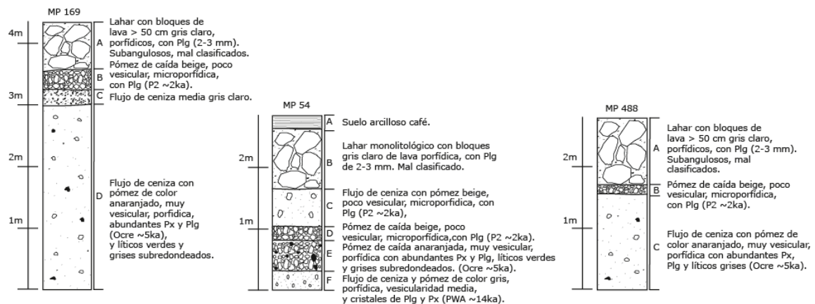
Figura. 38 Columnas estratigráficas que muestran la secuencia de los depósitos en la zona de Tehuixtlilán.
